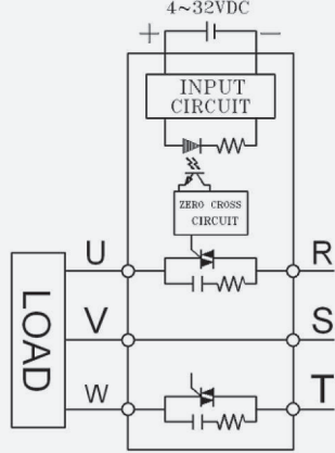
TSR-50DA-□ / TSR-75DA-□
